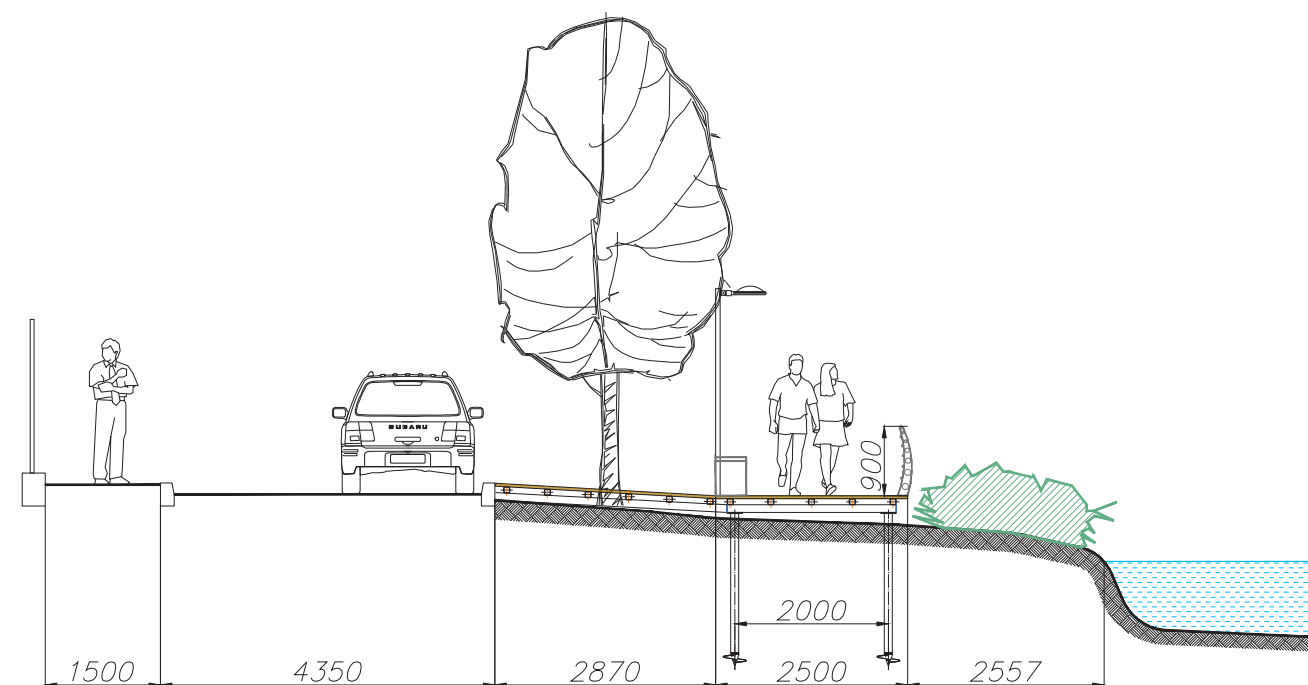
РАЗРЕЗ 2-2
