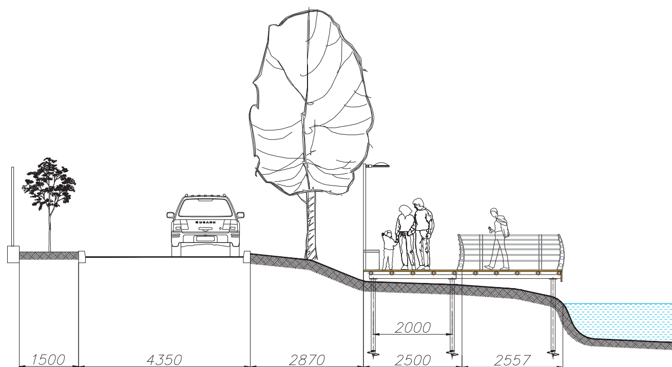
РАЗРЕЗ 1-1
